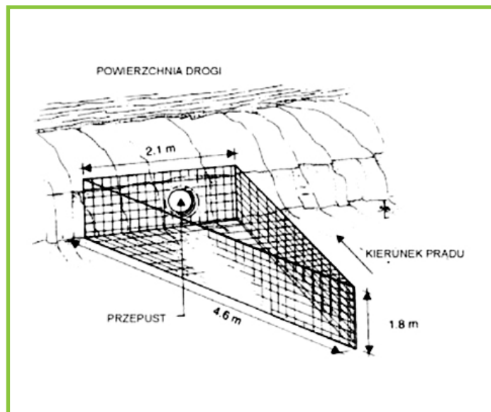
Rys. 2 Proste ogrodzenie przepustu.
